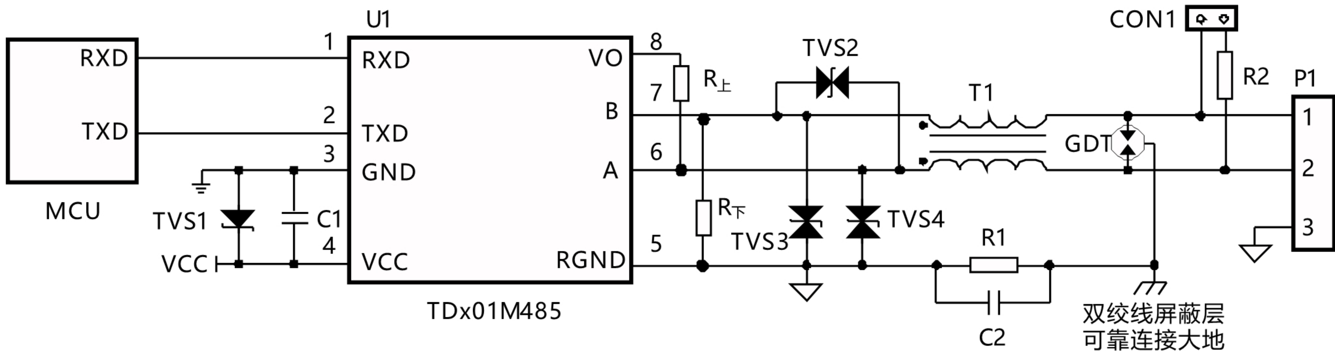
图3. EMC推荐电路
