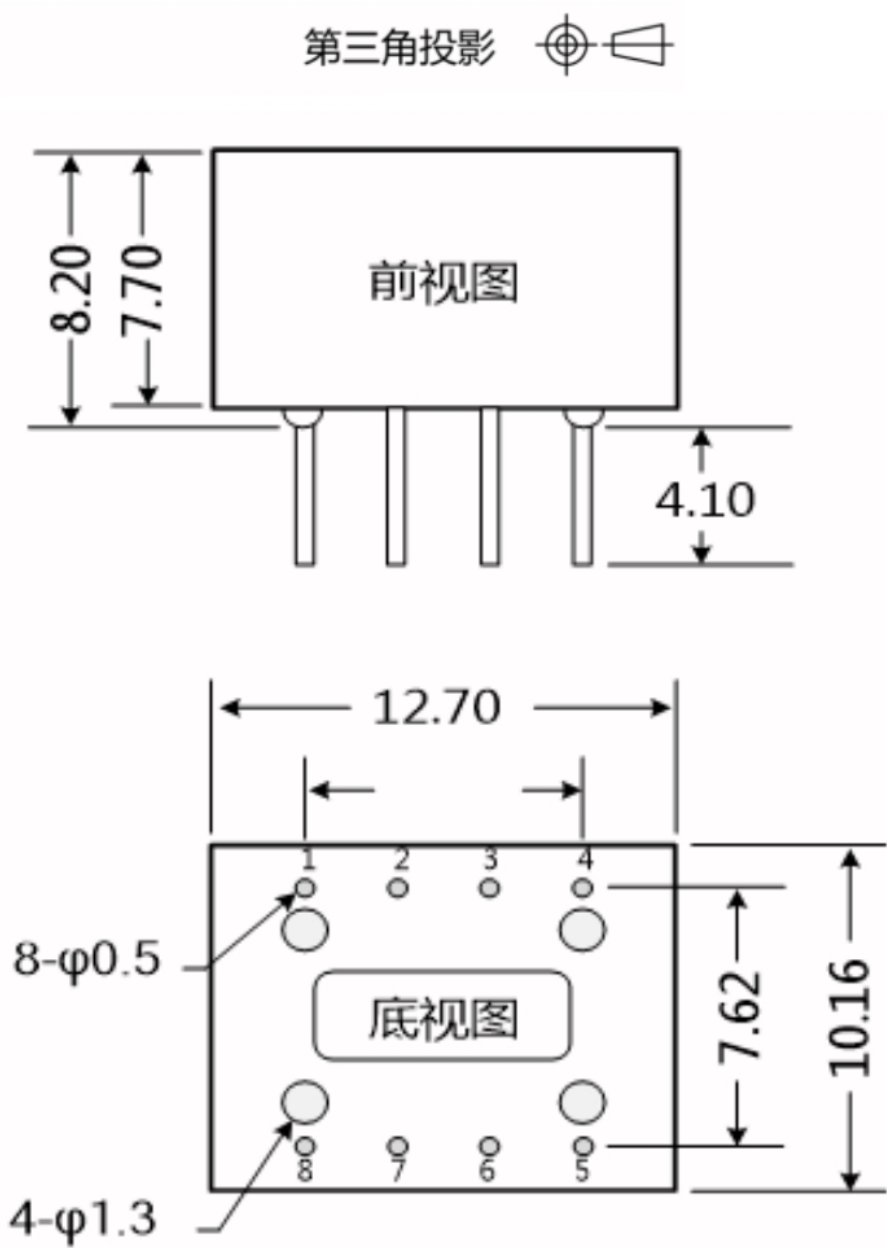
外观尺寸图
