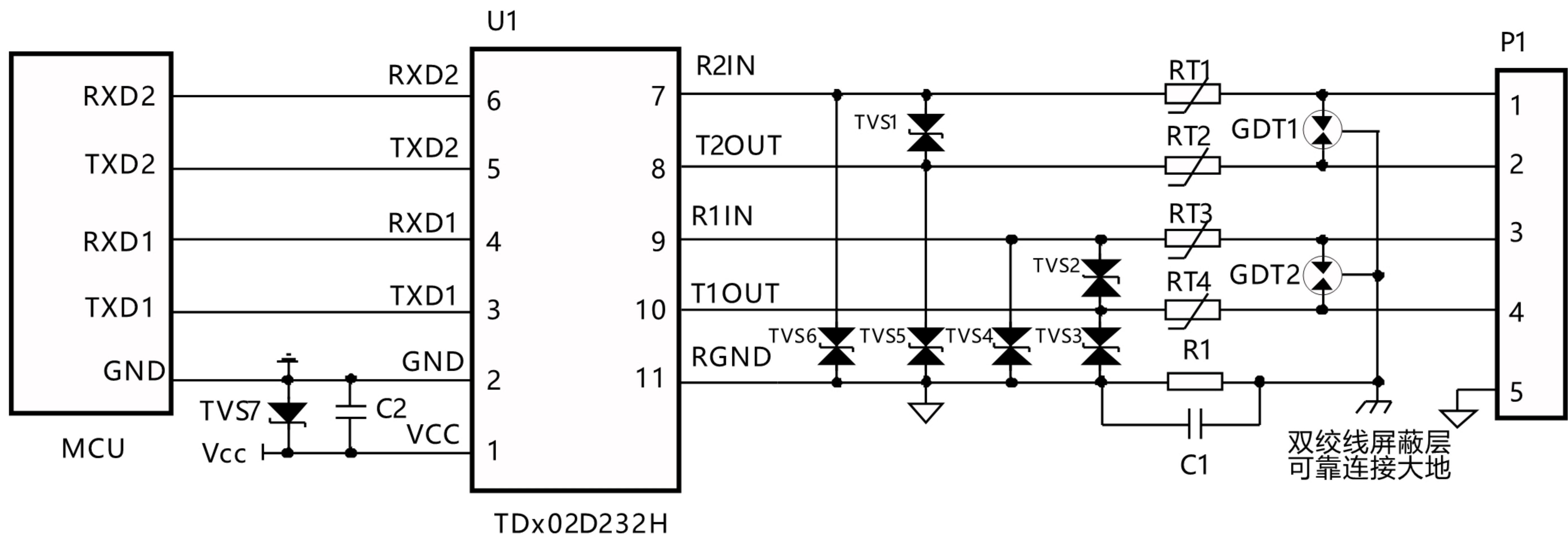
图2. EMC推荐电路
