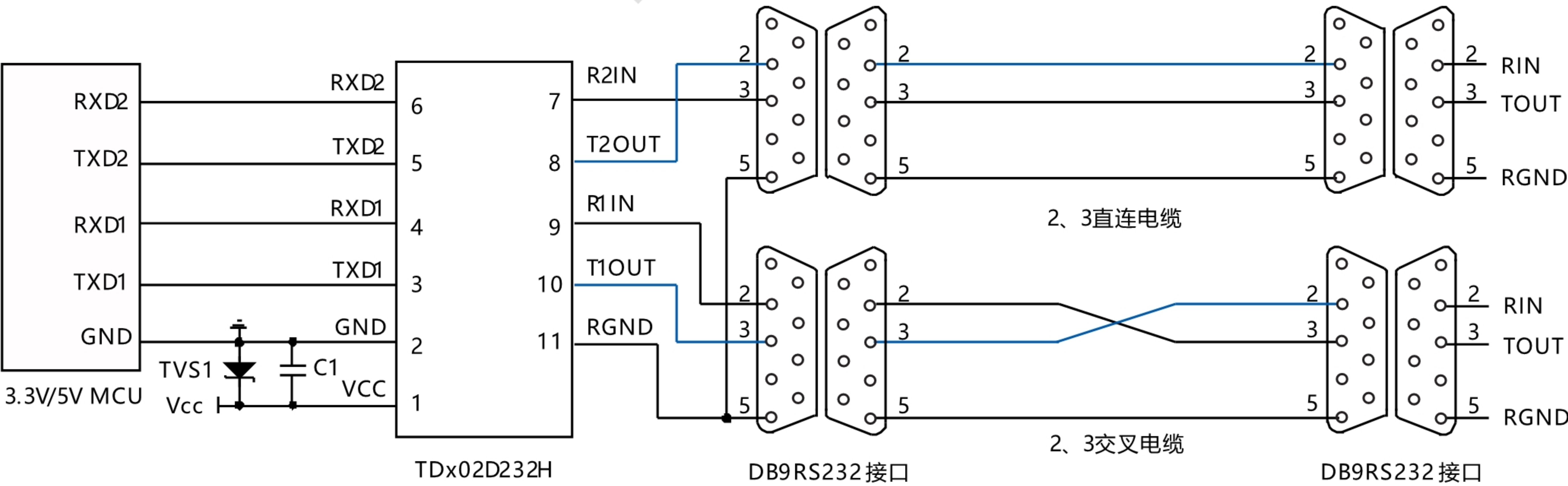
图 1. 典型连接电路图
