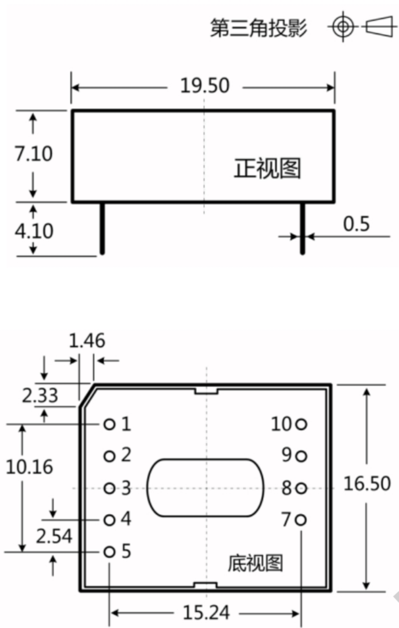
外观尺寸图
