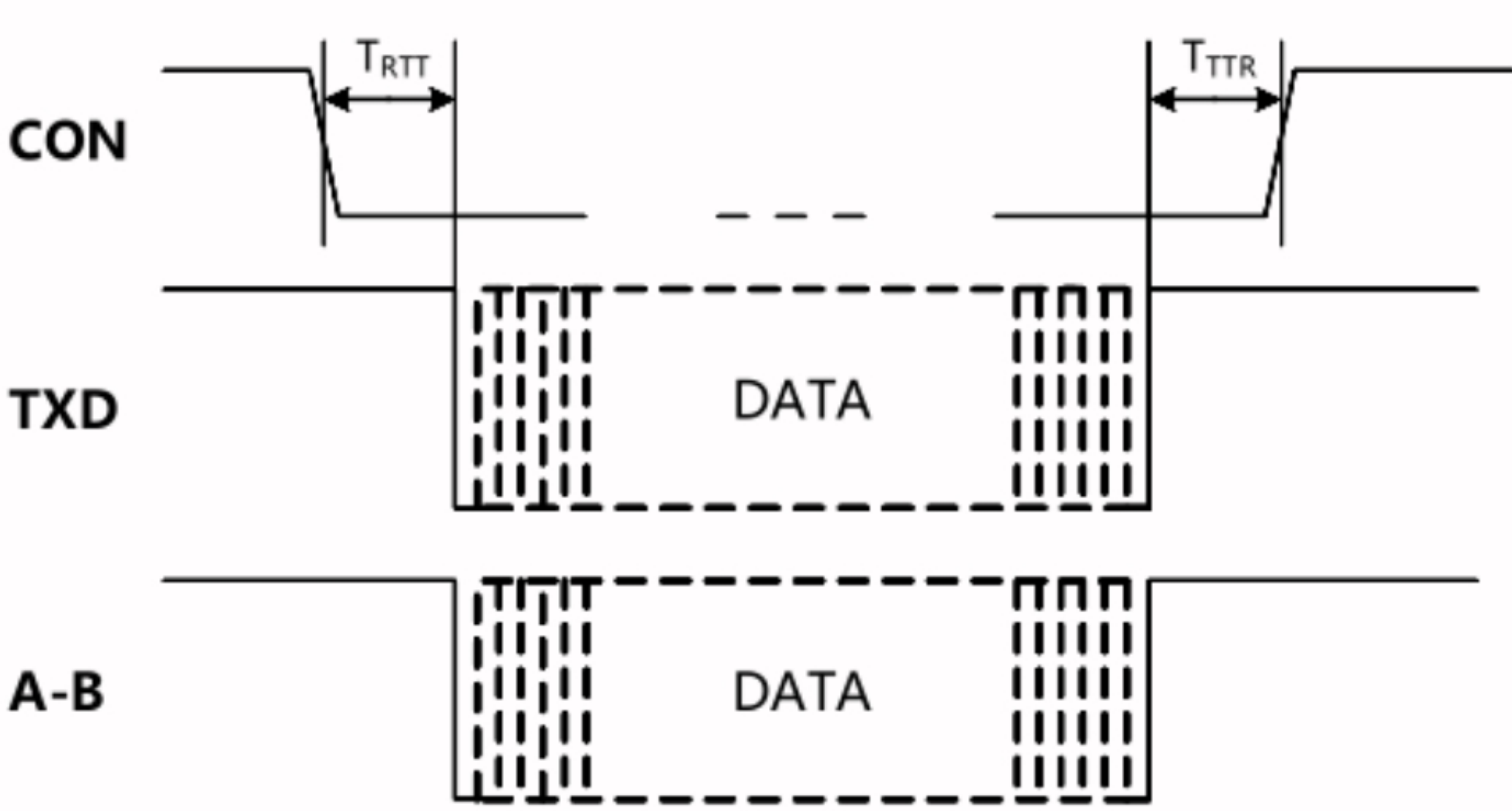
图1. TDx11D485模块数据发送时序图
