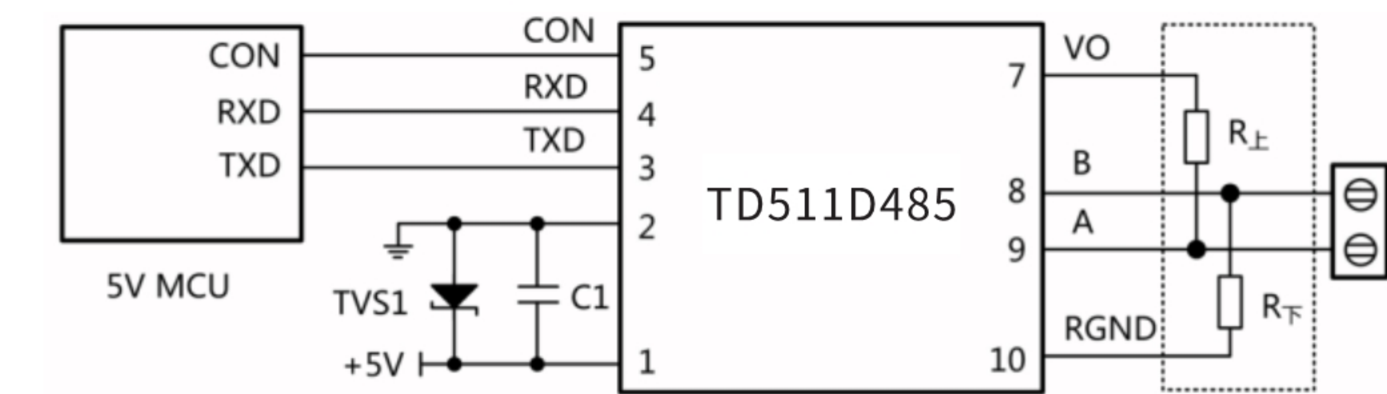
图3.MCU 5V供电应用电路
