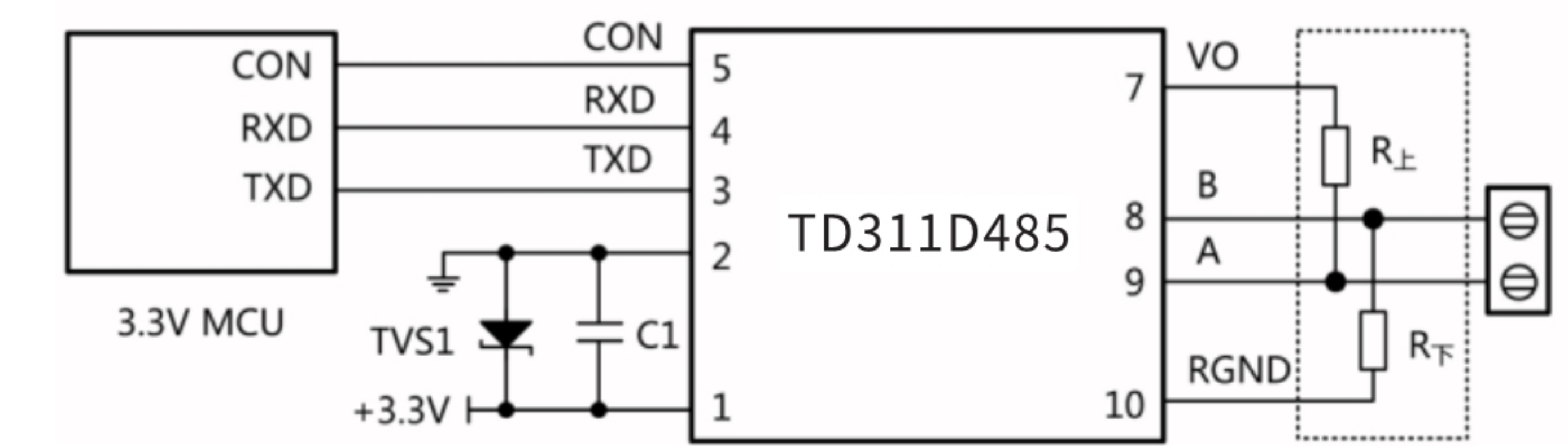
图4.MCU 3.3V供电应用电路
