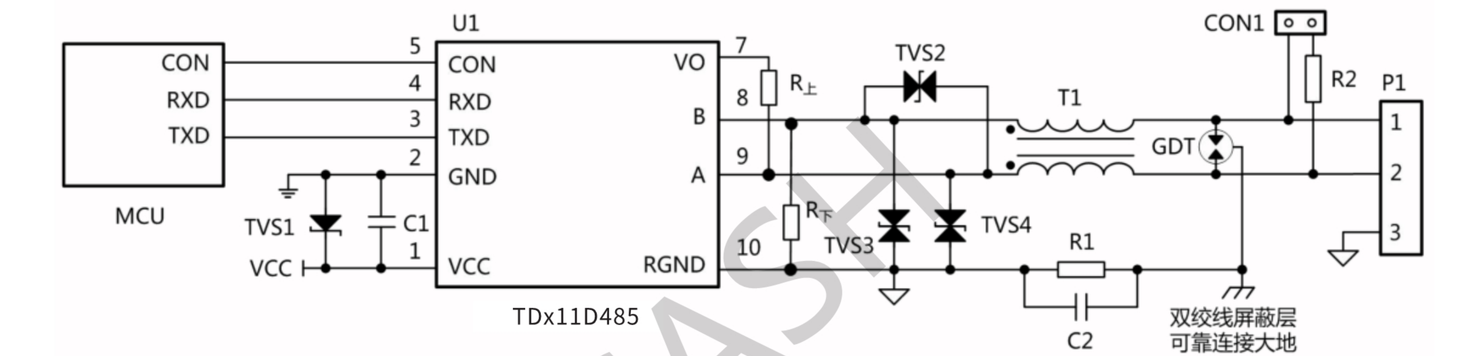
图5. EMC推荐电路
