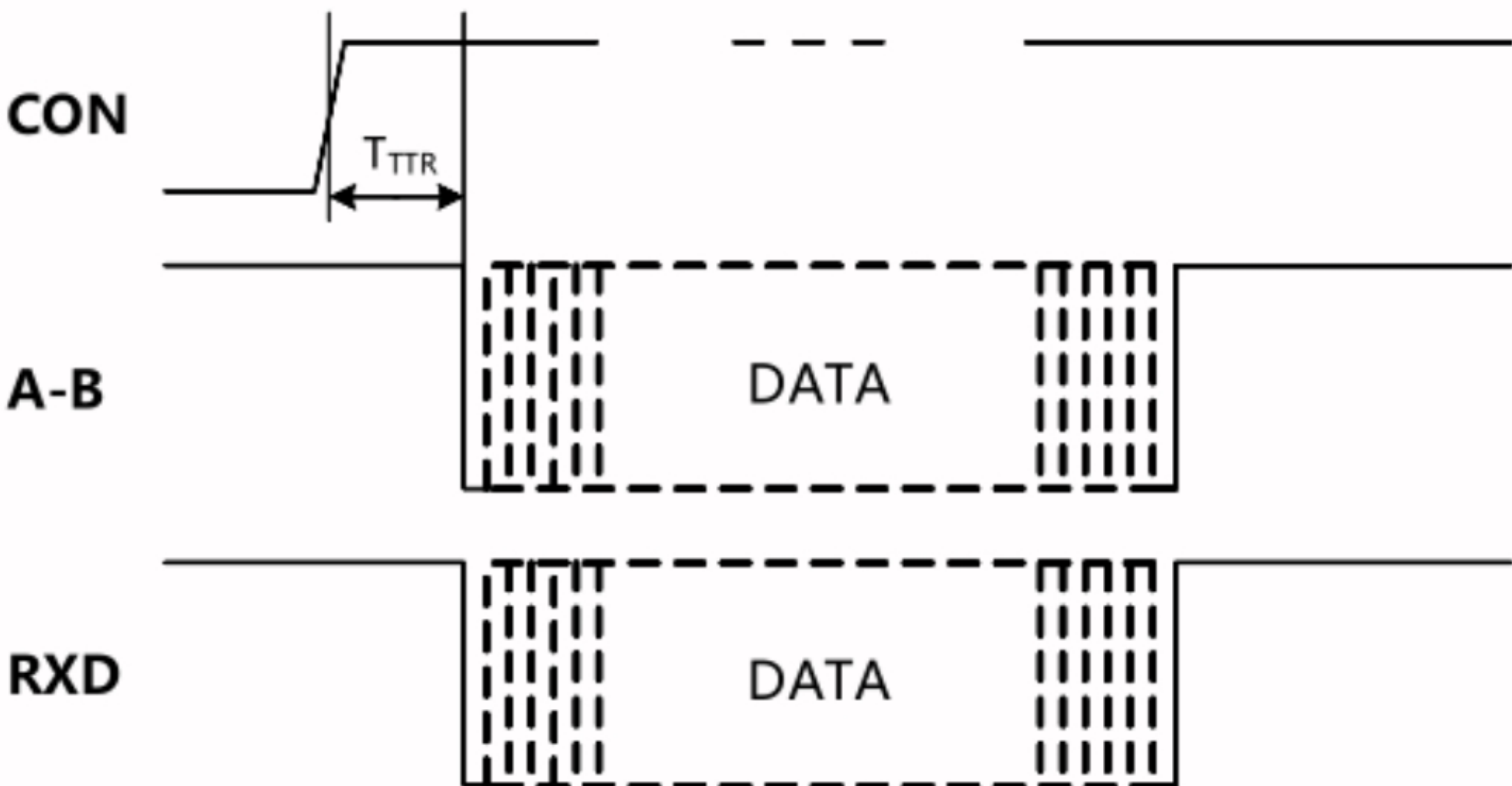
图2. TDx11D485模块数据接收时序图
