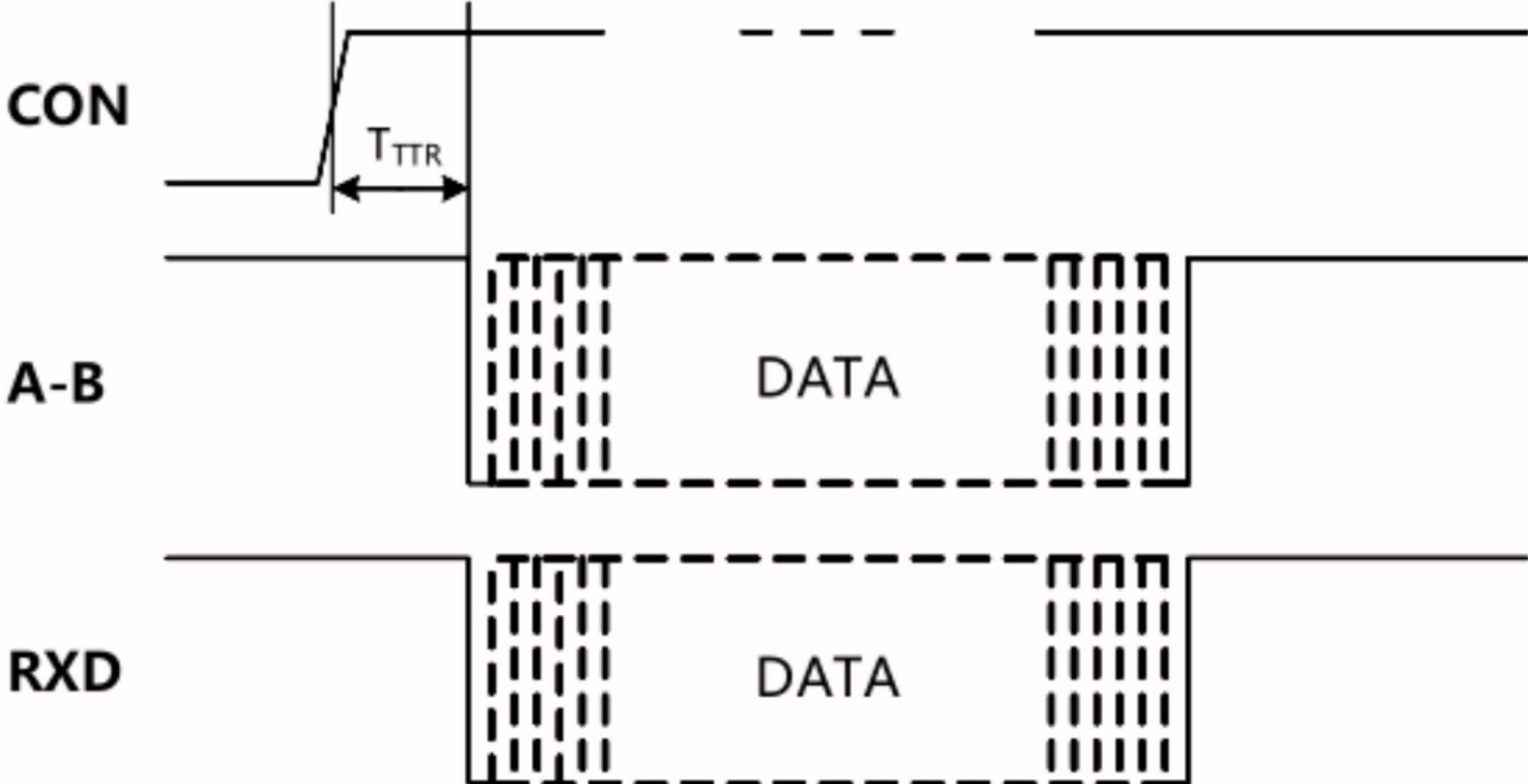
图 2. TDx11D485H模块数据接收时序图
