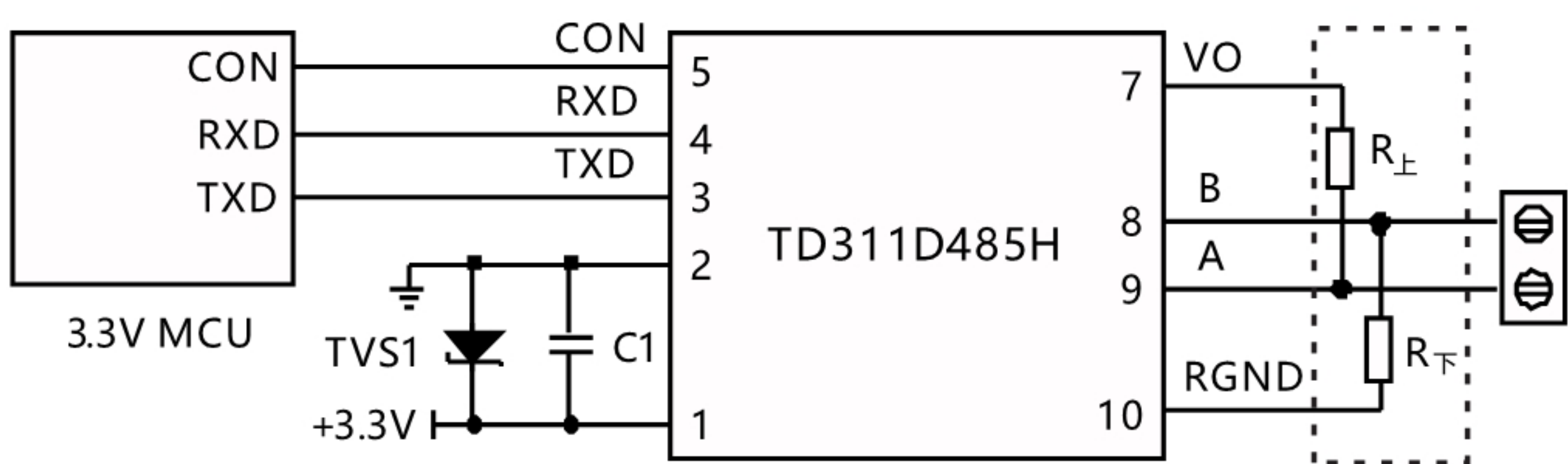
图4.MCU 3.3V供电应用电路
