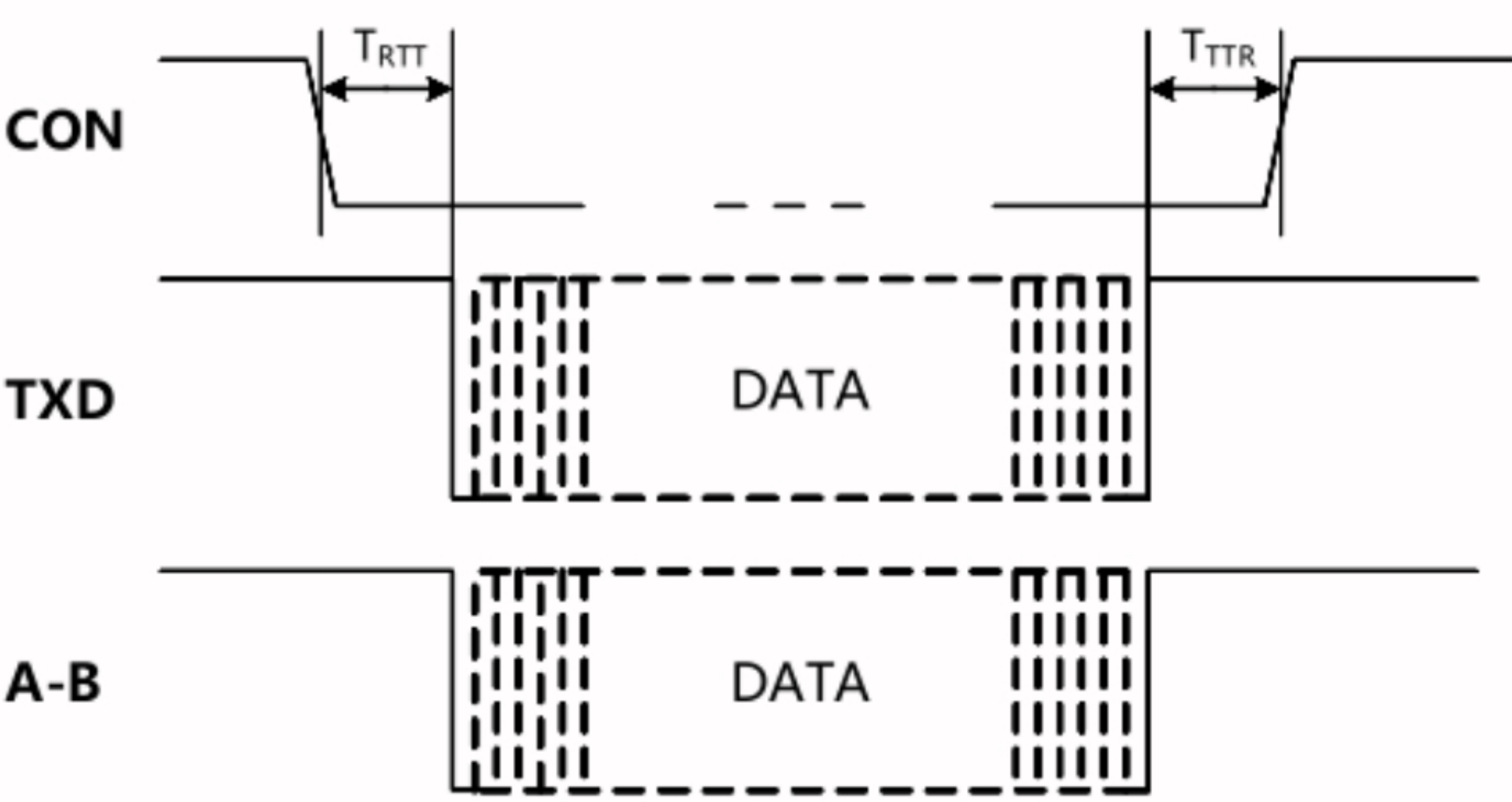
图 1. TDx11D485H模块数据发送时序图
