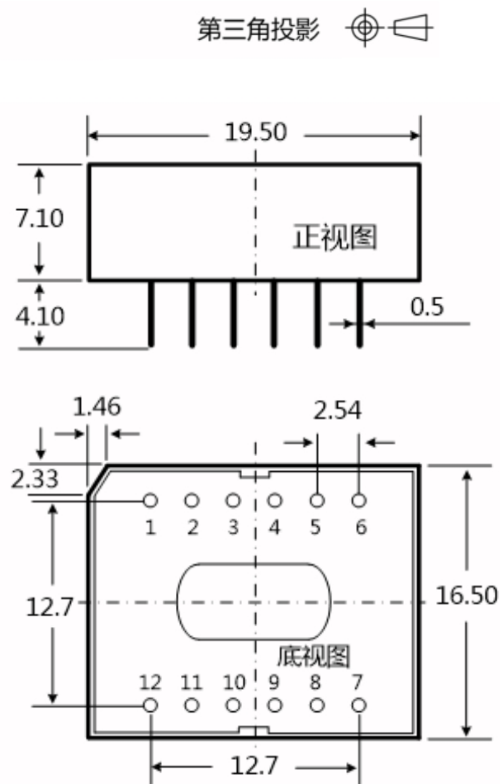
外观尺寸图
