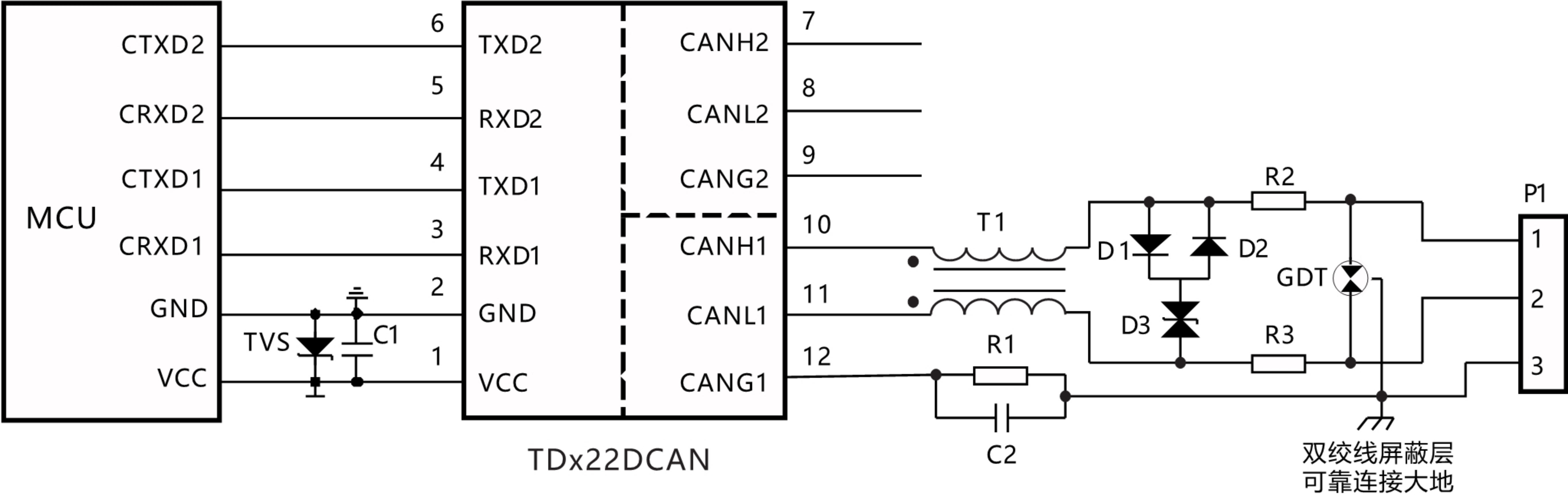
图2. EMC推荐电路
