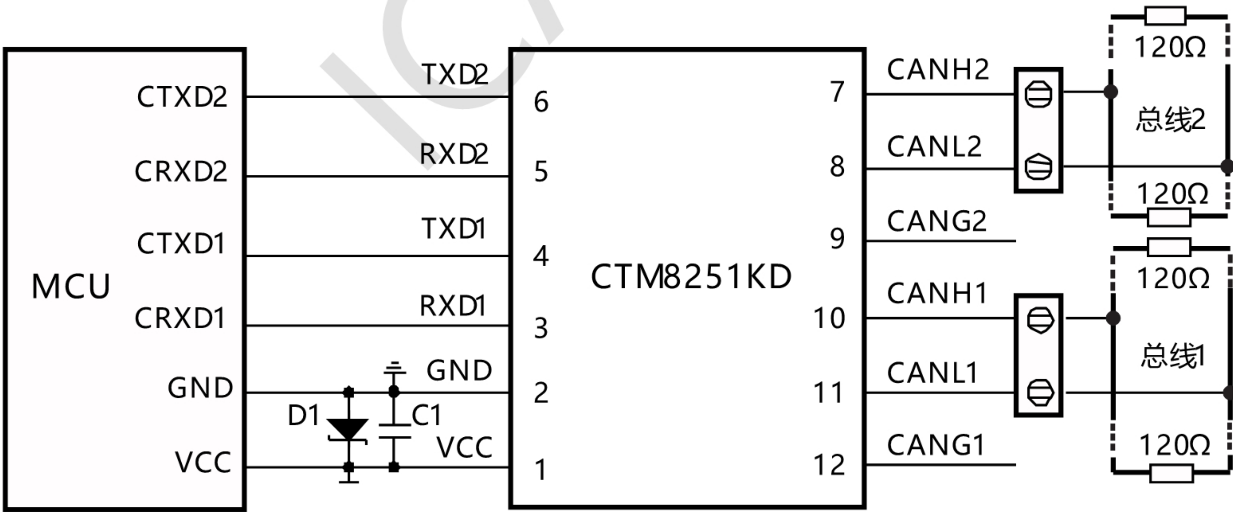
图 1.典型连接电路
