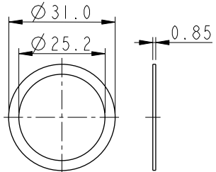
Gasket
